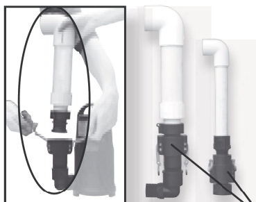
Комплект для подачи воды из насоса
