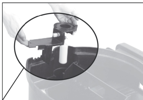
Система долива Auto-fill
